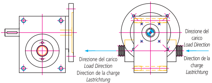
Forma 14 / Type 14 / Forme 14 / Bauart 14
